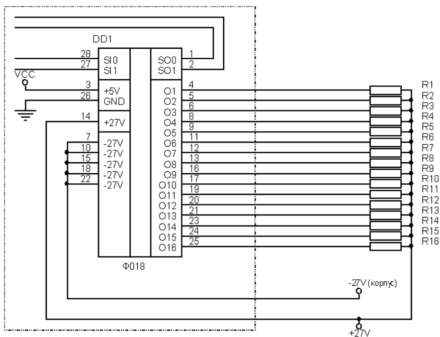
Типовая схема включения микросборки Ф018
