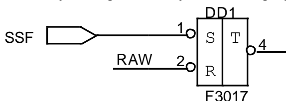
Рисунок 6.4 – триггер фиксации разрядов ОС
