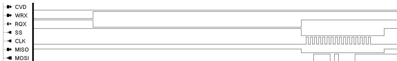
Рисунок 6.2 – диаграмма сигналов при передаче из подсистемы пользователя слова данных
