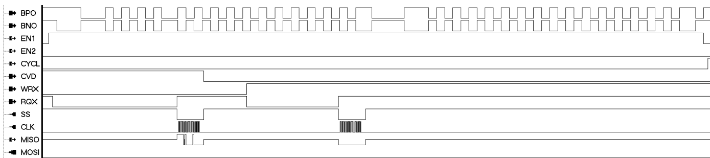
Рисунок 6.3 - диаграмма приема КС и выдачи первого СД
