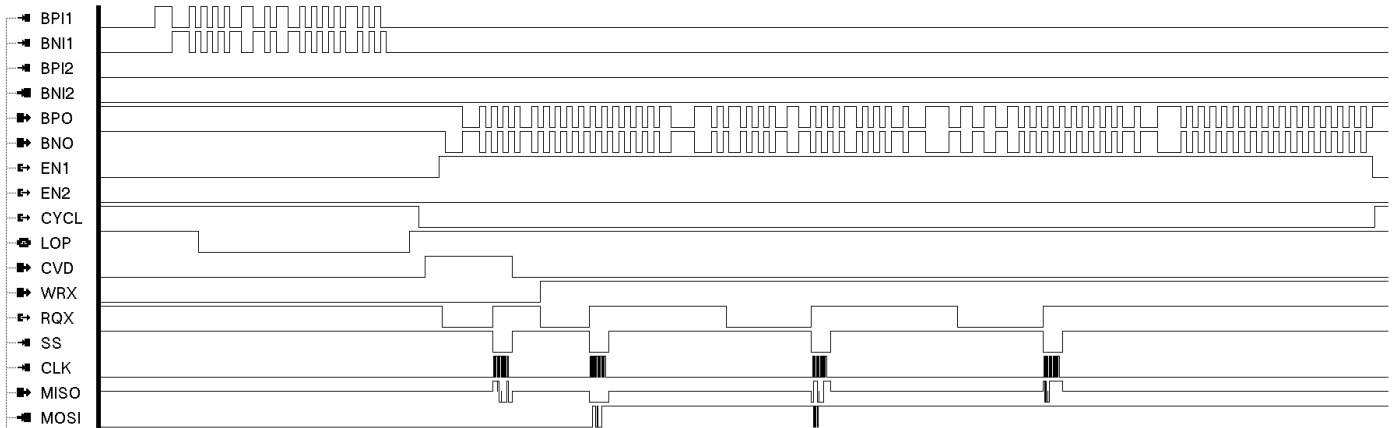
Рисунок 6.1 – диаграмма сигналов при приеме КС «Передать 3 слова данных»
