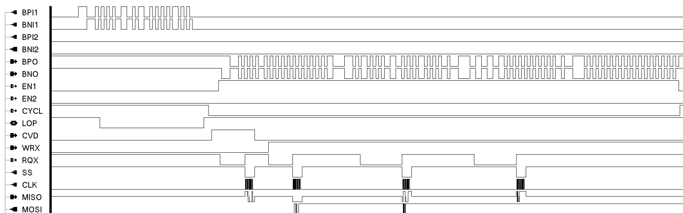
Рисунок 6.1 – диаграмма сигналов при приеме КС «Передать 3 слова данных»
